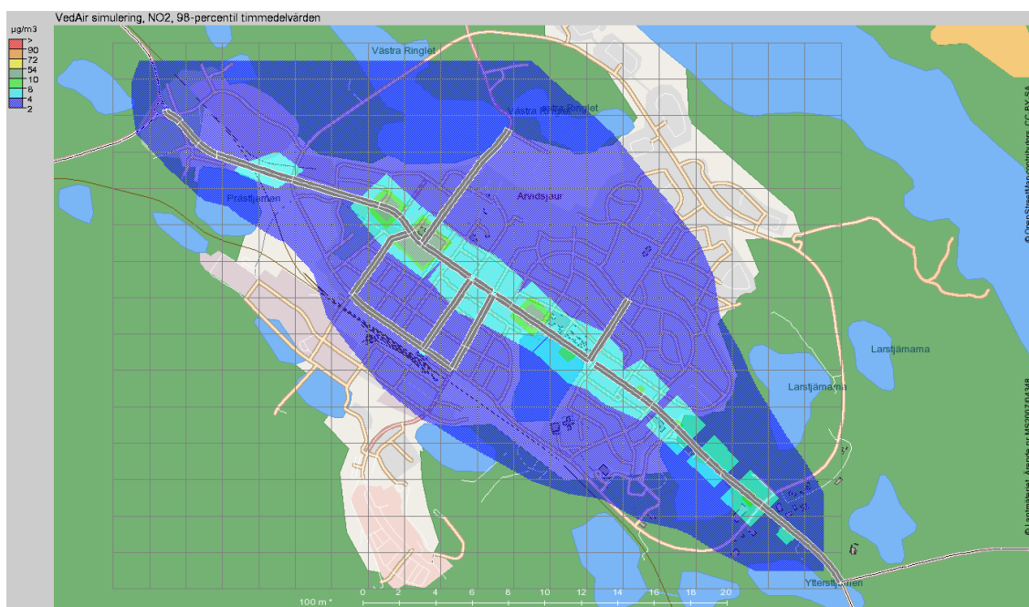
Figur 5: 98-percentil av timmedelhalt av NO 2 för Arvidsjaur's tätort.
