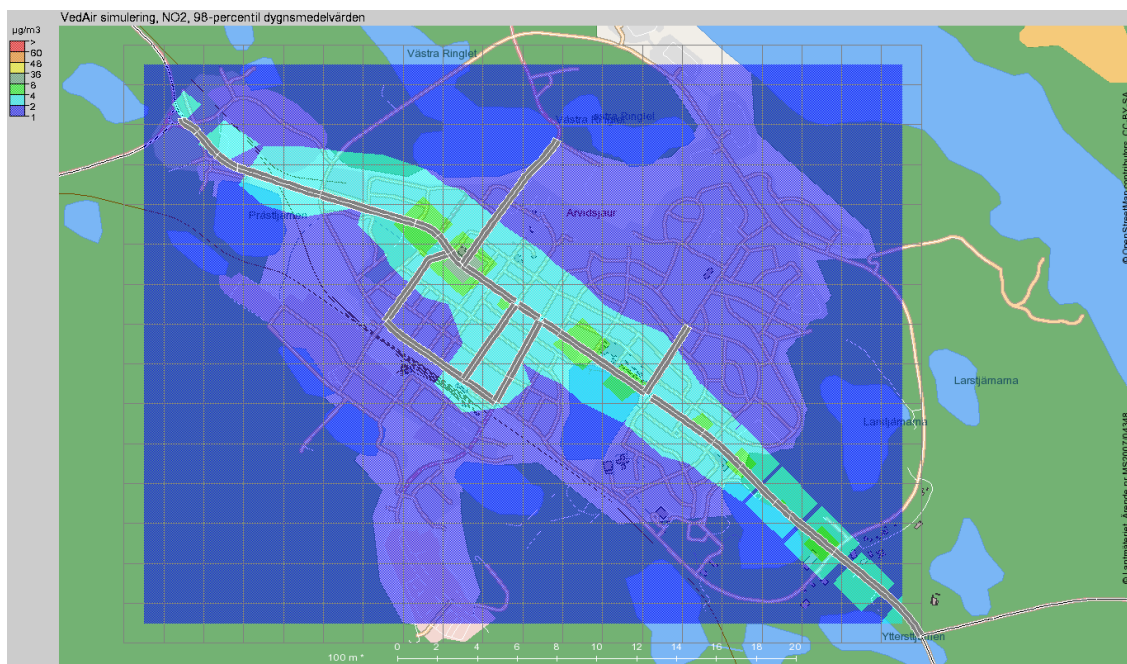
Figur 4: 98-percentil av dygnsmedelhalt av NO 2 för Arvidsjaur tätort.
