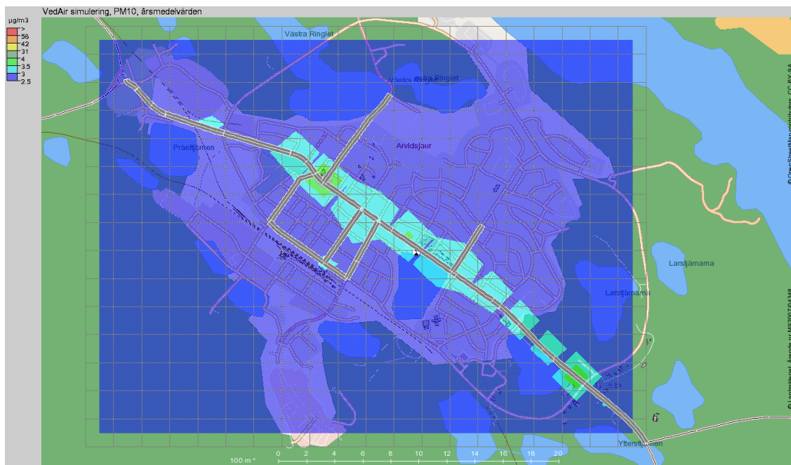
Figur 1: Årsmedelhalt av PM10 för Arvidsjaur tätort.
