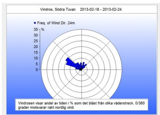
Figur 9. Vindros för v.8 år 2013
