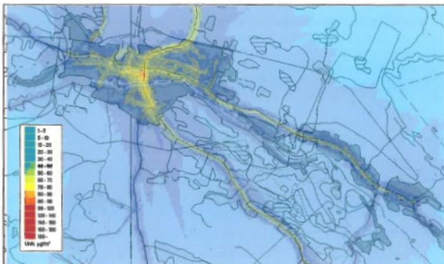
Figur 4.1.3 Beräknad 98-percentil (timme) av NO 2 -halter. MKN = 108 µg/m 3 (inklusive toleransmarginal för år 2002)
