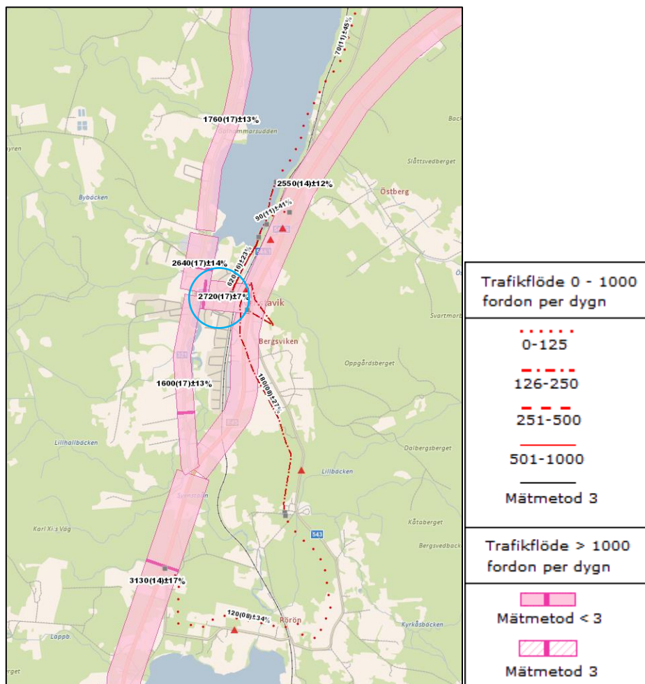
Figur 2 - Trafikflödesmätningar i och kring Svenstavik 2018. Den blå cirkeln visar området för beräkningar
