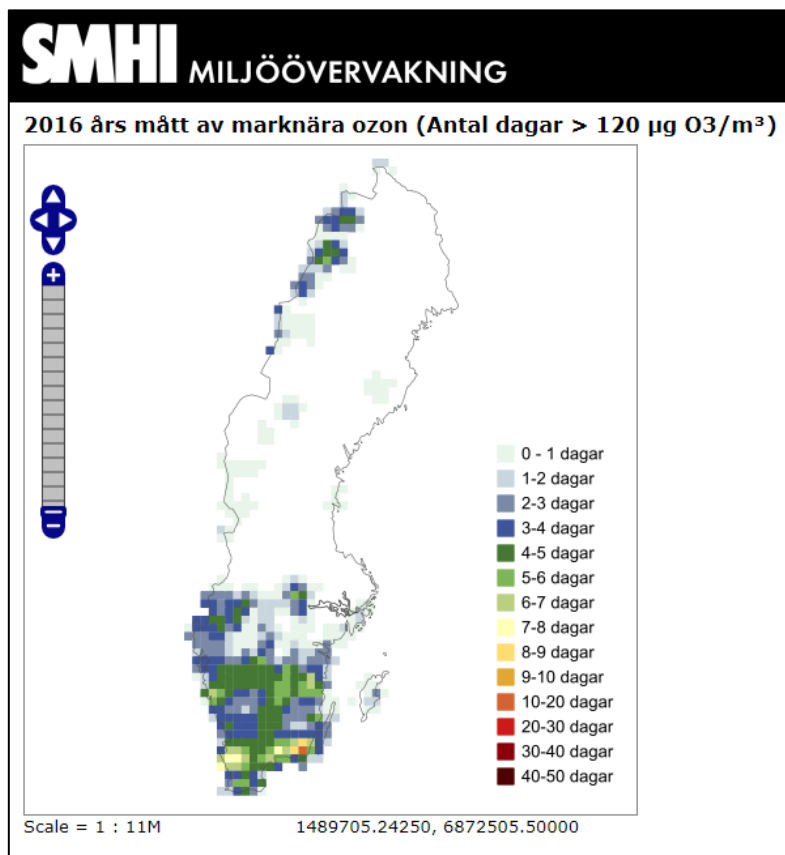
Figur 1 - Kartbild över mått av marknära ozon 2016
