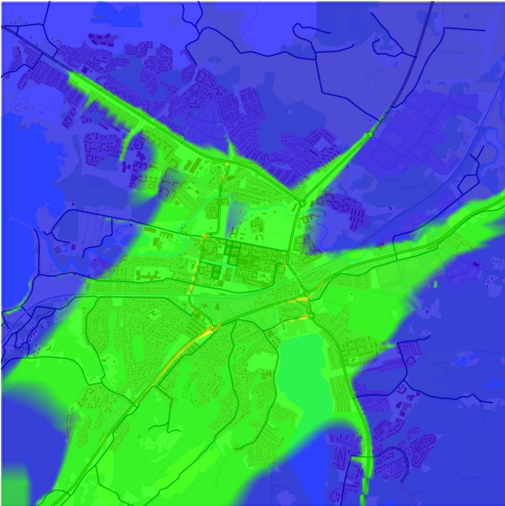
Figur 3. Beräknat timmedelvärde (98-percentil) för kvävedioxidhalter i tätortsområdet Alingsås i Alingsås kommun år 2015.
