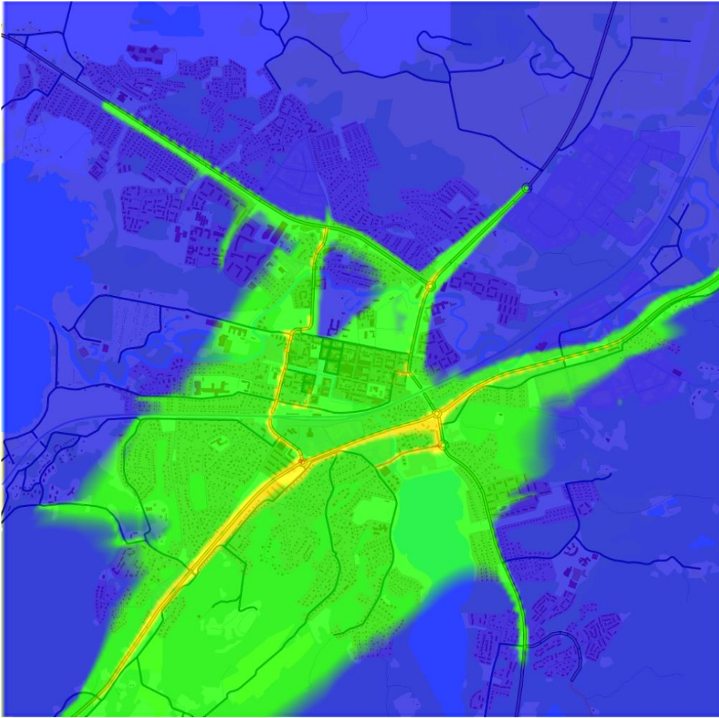
Figur 2. Beräknat dygnsmedelvärde (98-percentil) för kvävedioxidhalter i tätortsområdet Alingsås i Alingsås kommun år 2015.
