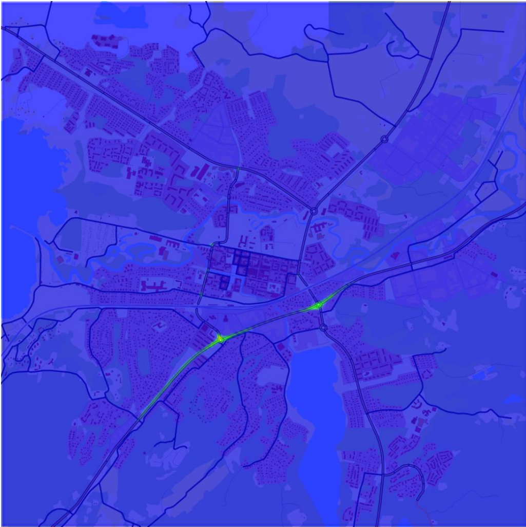
Figur 1. Beräknat årsmedelvärde för kvävedioxidhalter i tätortsområdet Alingsås i Alingsås kommun år 2015.
