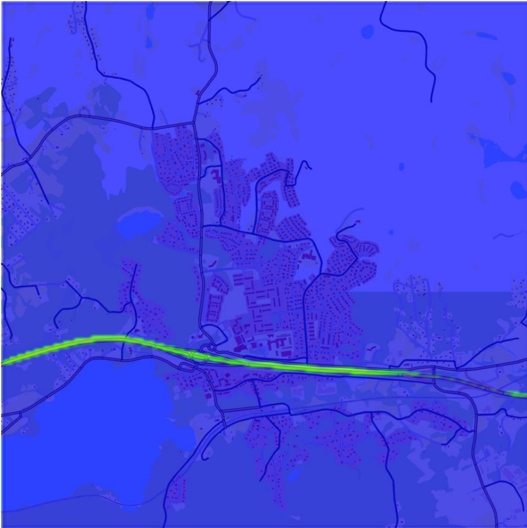
Figur 1. Beräknat årsmedelvärde för kvävedioxidhalter i Landvetter tätort i Härryda kommun år 2015.
