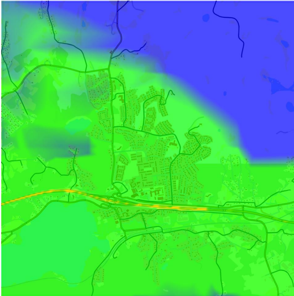
Figur 3. Beräknat timmedelvärde (98-percentil) för kvävedioxidhalter i Landvetter tätort i Härryda kommun år 2015.
