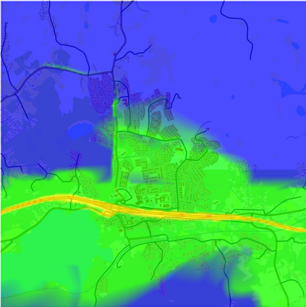
Figur 2. Beräknat dygnsmedelvärde (98-percentil) för kvävedioxidhalter i Landvetter tätort i Härryda kommun år 2015.
