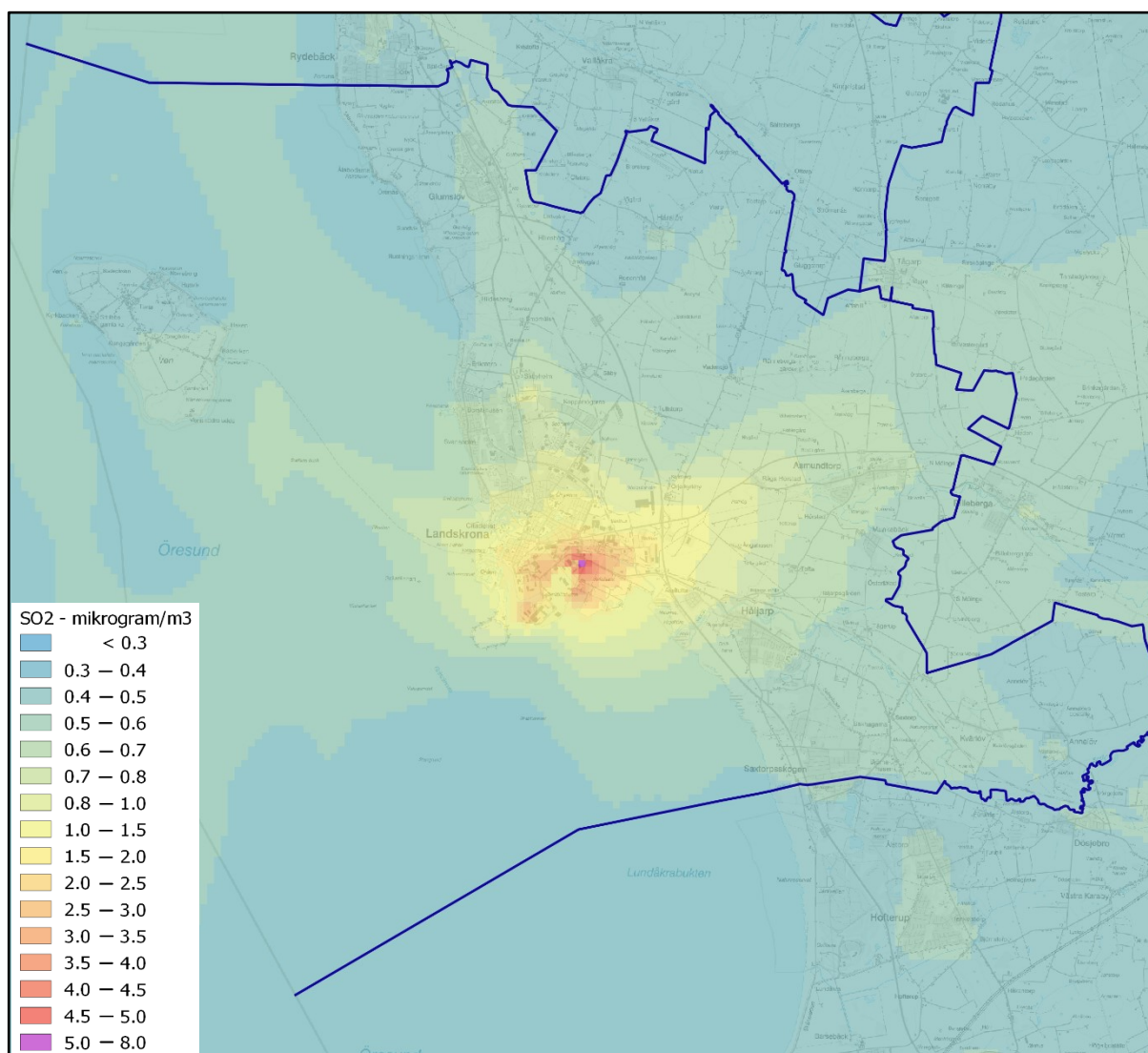
Figur 3. Beräknade halter av årsmedelvärde för svaveldioxid (SO 2 ) inom Landskrona kommun år 2019.
