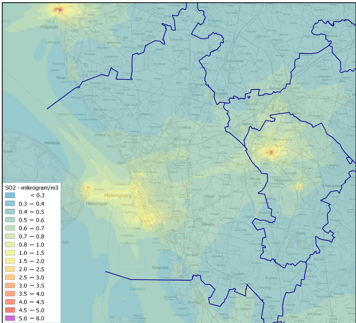
Figur 4. Beräknade halter av årsmedelvärde för svaveldioxid (SO 2 ) inom Helsingborg och Bjuvs kommun år 2019.
